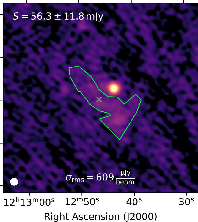
NGC 4178 / IC 3042 / VCC 66
